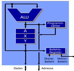
Prozessor
